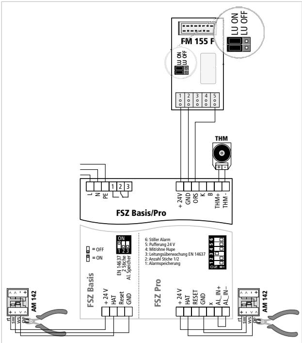
Abb. 15: Funkbetrieb mit Leitungüberwachung
