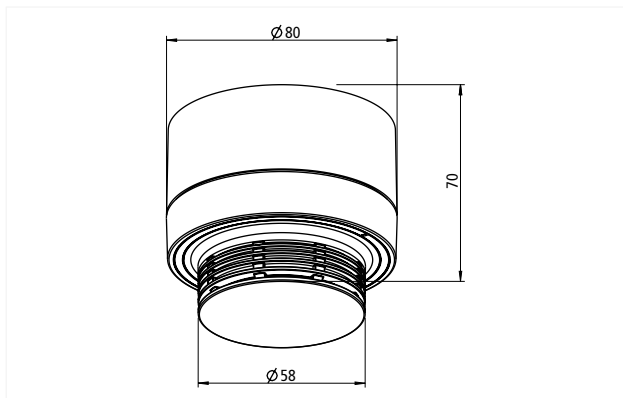
Abb. 11: Maßzeichnung
